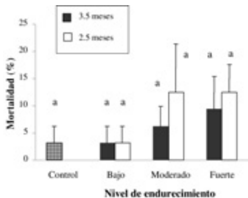
Figura 2. Mortalidad de plántulas de Quercus ilex al año de ser plantados en ambiente xérico según los niveles de endurecimiento
