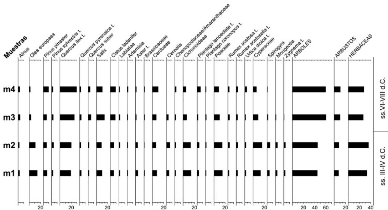
Figura 2. Diagrama palinológico del yacimiento de El Saucedo
