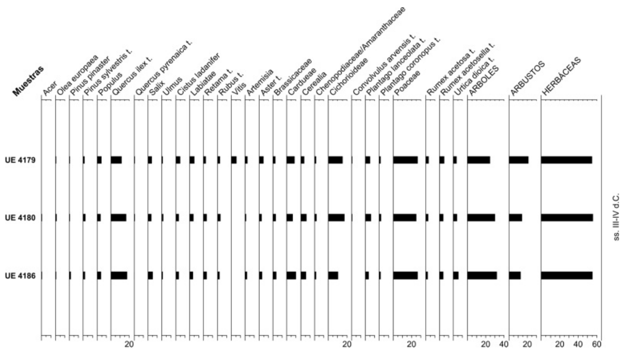
Figura 1. Diagrama palinológico del yacimiento de Carranque
