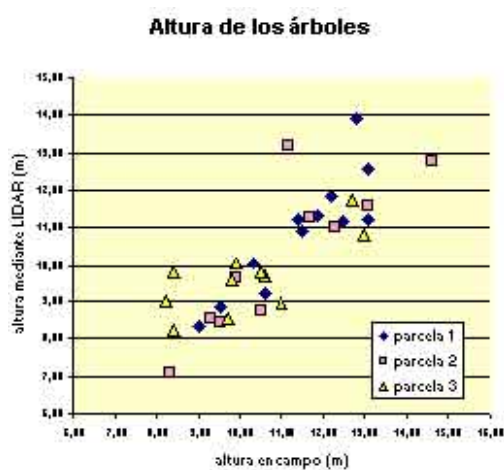
Fig. 2: Relación entre la altura total medida en campo con la altura a partir de datos lidar (m)
