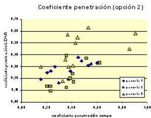
Figura 4: Relación entre el coeficiente de penetración medido en campo respecto la medición con datos lidar (opción 2)
