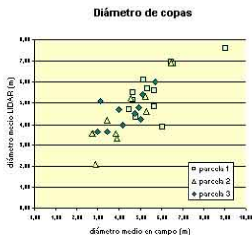
Fig. 3: Relación entre el diámetro medio medido en campo con el diámetro medio a partir de datos lidar (m)
